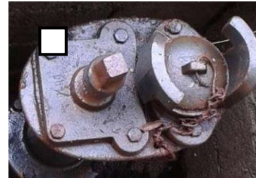
Chiave quadra per idranti sottosuolo ch 27÷30
