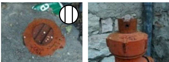
Slot 25 (manico chiave manichette), chiave manichette 100/70, Chiave sagomata, chiave a settore con nasello \varnothing max 8 o a mano
